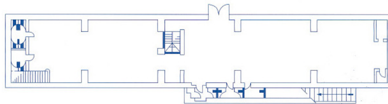
PIANTA PIANO TERRA
